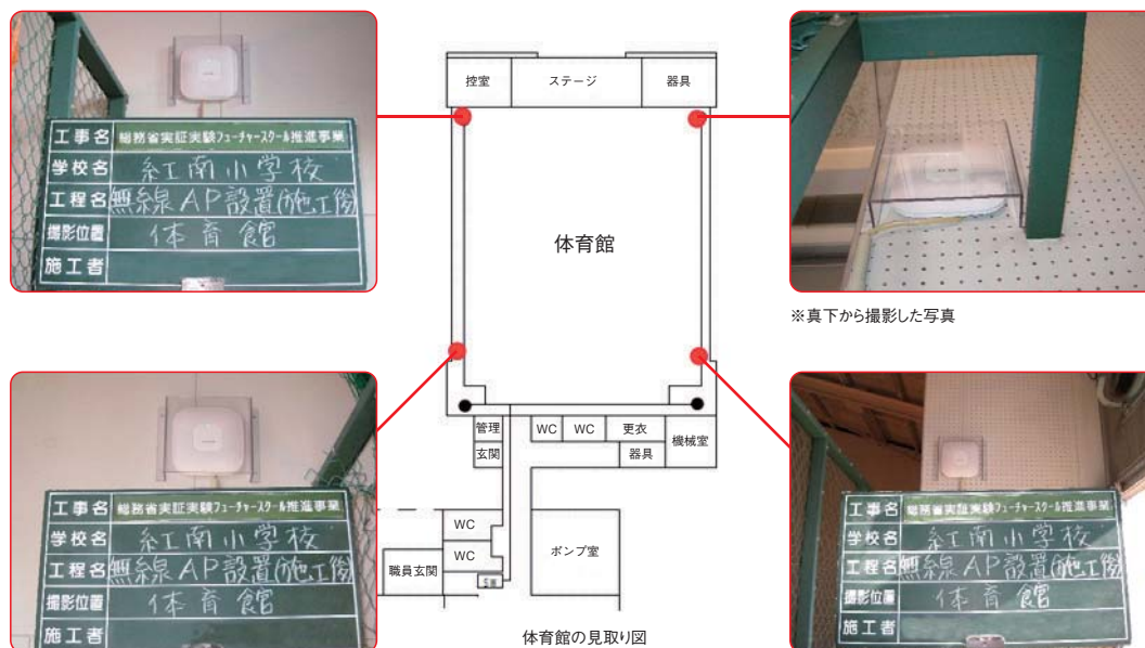
体育館の四隅付近の壁にアクセスポイントを4基設置した例
